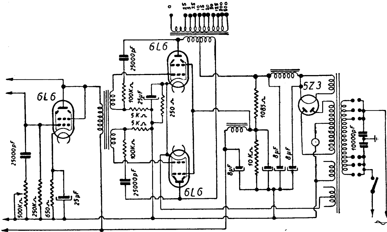
WATT RADIO - Mod. AUDITORIUM JUNIOR - In alto schema AF/MF, in basso amplificatore finale. Classe AB2. Media frequenza 470 kc.
